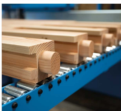
UITSPARINGEN FREZEN
